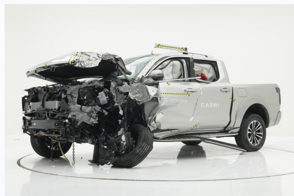
> 驾驶员侧正面25%偏置碰撞
